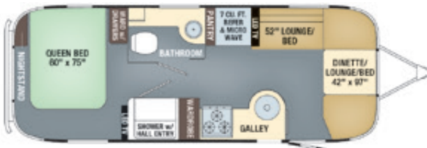
25RB
